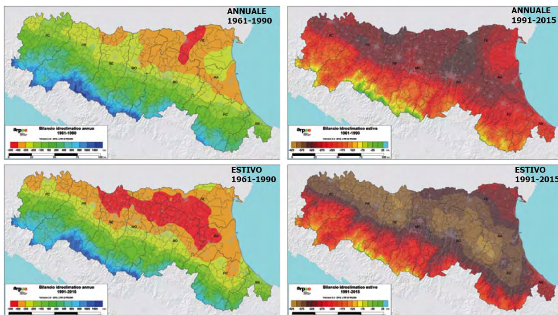
Figura 18 - Confronto bilancio idroclimatico (BIC) annuo ed estivo (precipitazioni - etp)
