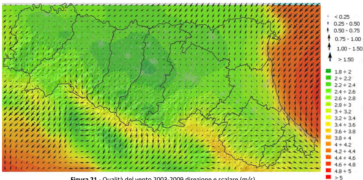
Figura 21 - Qualità del vento 2003-2009 direzione e scalare (m/s)
