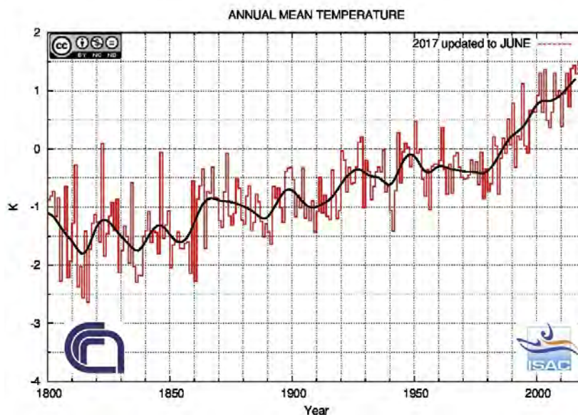
Figura 3- Variazione temperatura media annua dal 1800 in Italia
